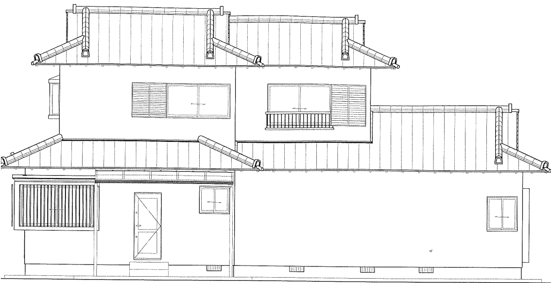
南側 立面図 S:1/100
