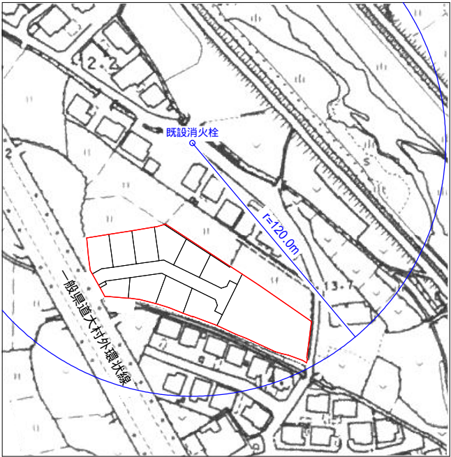
既設消火栓位置図 S=1:2500
